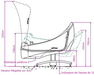
CUVE EN POSITION HAUTE AVEC PIÉTEMENT
