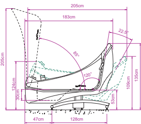
CUVE EN POSITION BASSE AVEC PIÉTEMENT
