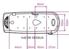
CUVE EN POSITION HAUTE AVEC PIÉTEMENT
