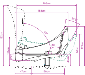
CUVE EN POSITION BASSE SANS PIÉTEMENT
