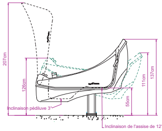
CUVE EN POSITION HAUTE SANS PIÉTEMENT
